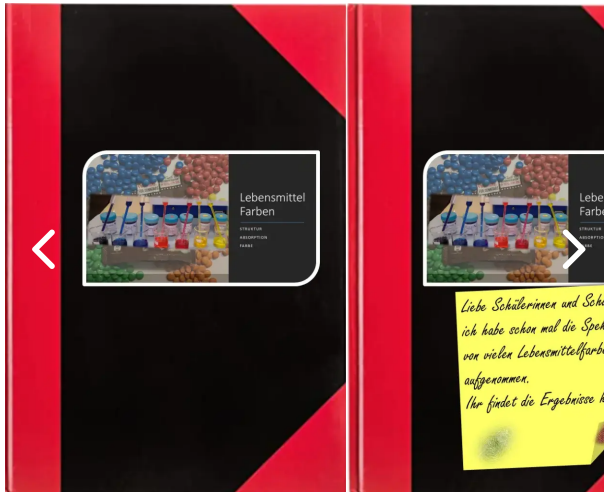
Abb. 1: Farbigkeit und Absorptionsspektren diverser Lebensmittelfarben 1
