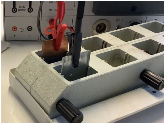
Abb. 1: Experimenteller Aufbau.
