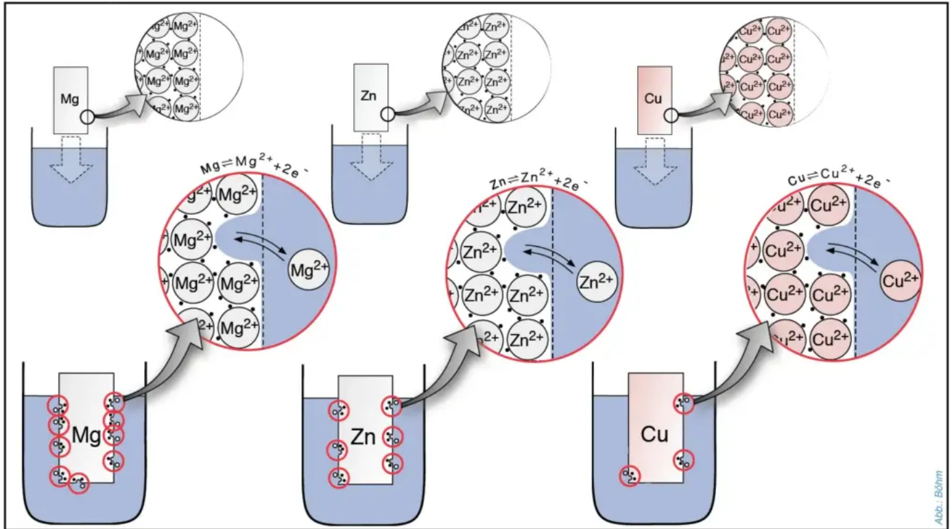
Abb. 1: Modell zur Lösungstension und zur elektrochemischen Doppelschicht.
